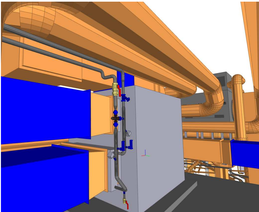
Vue de la centrale de traitement d'air à installer
